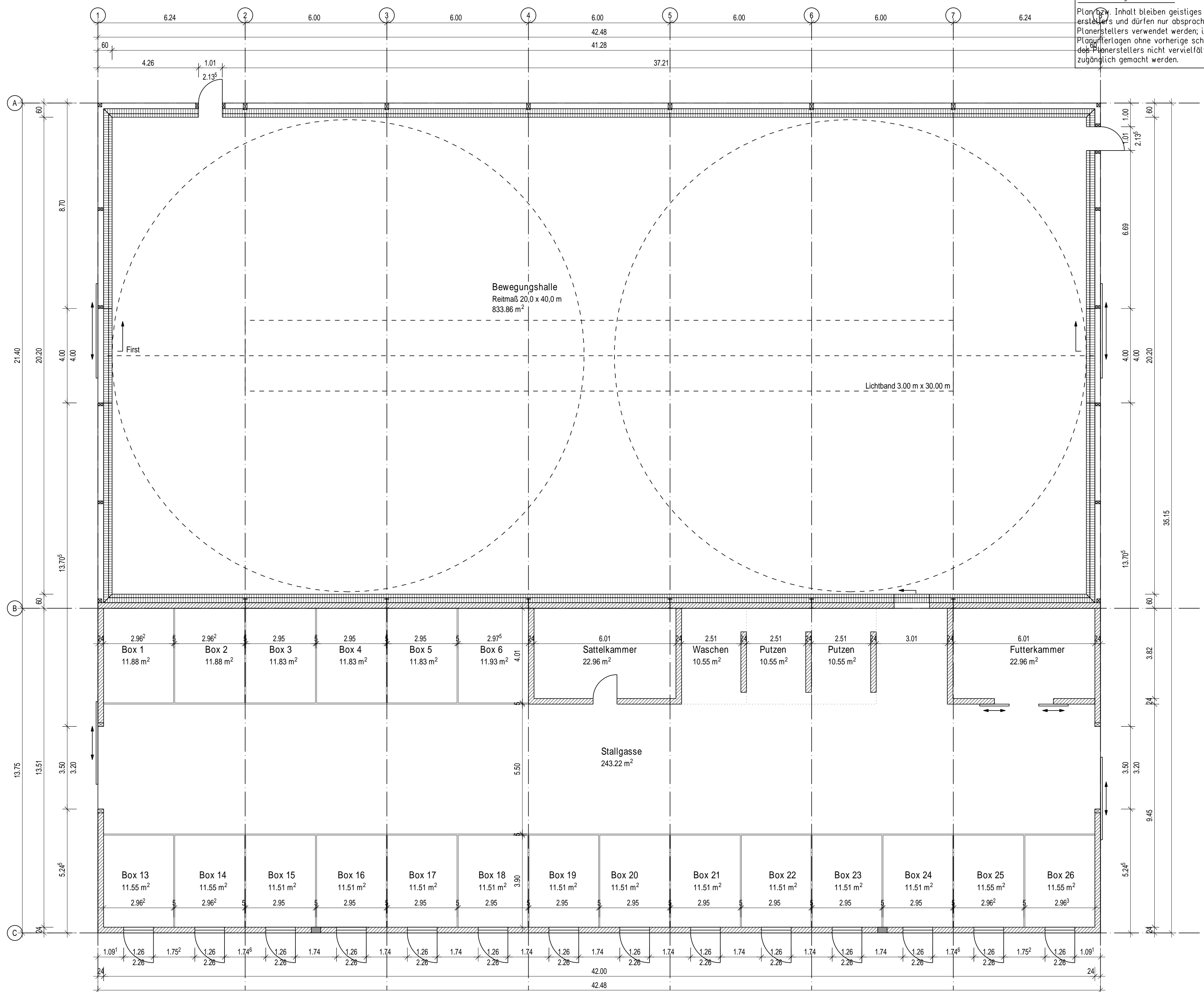
Grundriss
