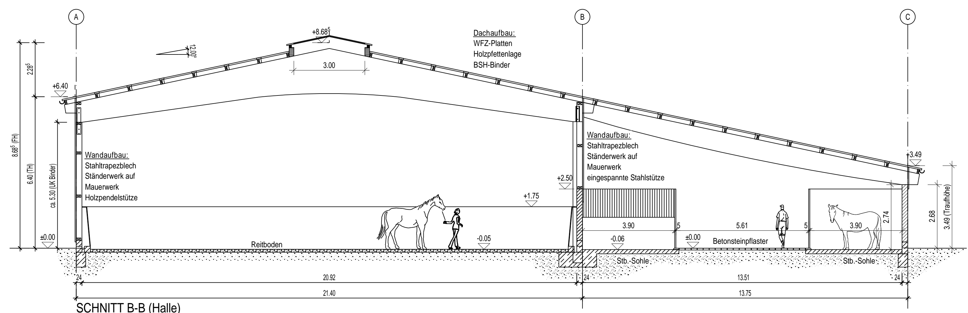
SCHNITT B-B (Halle)
